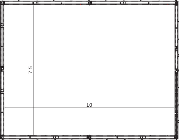
Bovenaanzicht + binnenmaten
