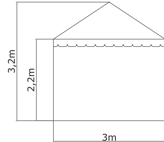
Doorsnede + binnenmaten
